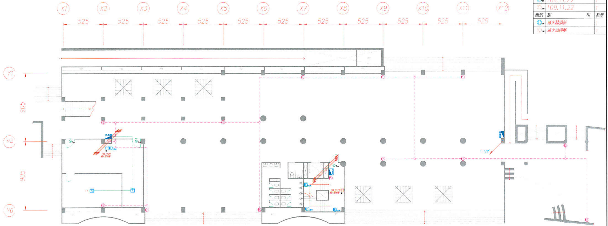
迎曦樓壹樓消防平面圖
