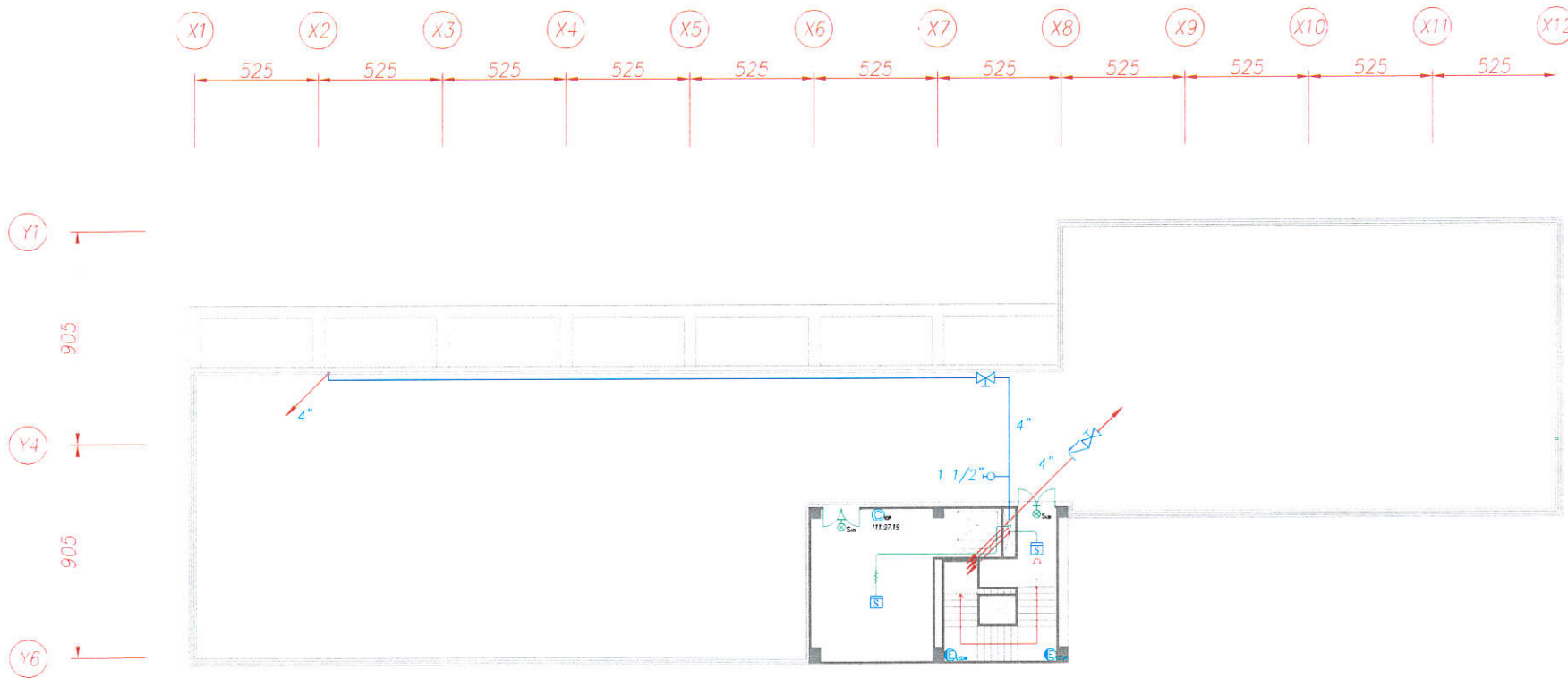
迎曦樓頂樓消防平面圖
