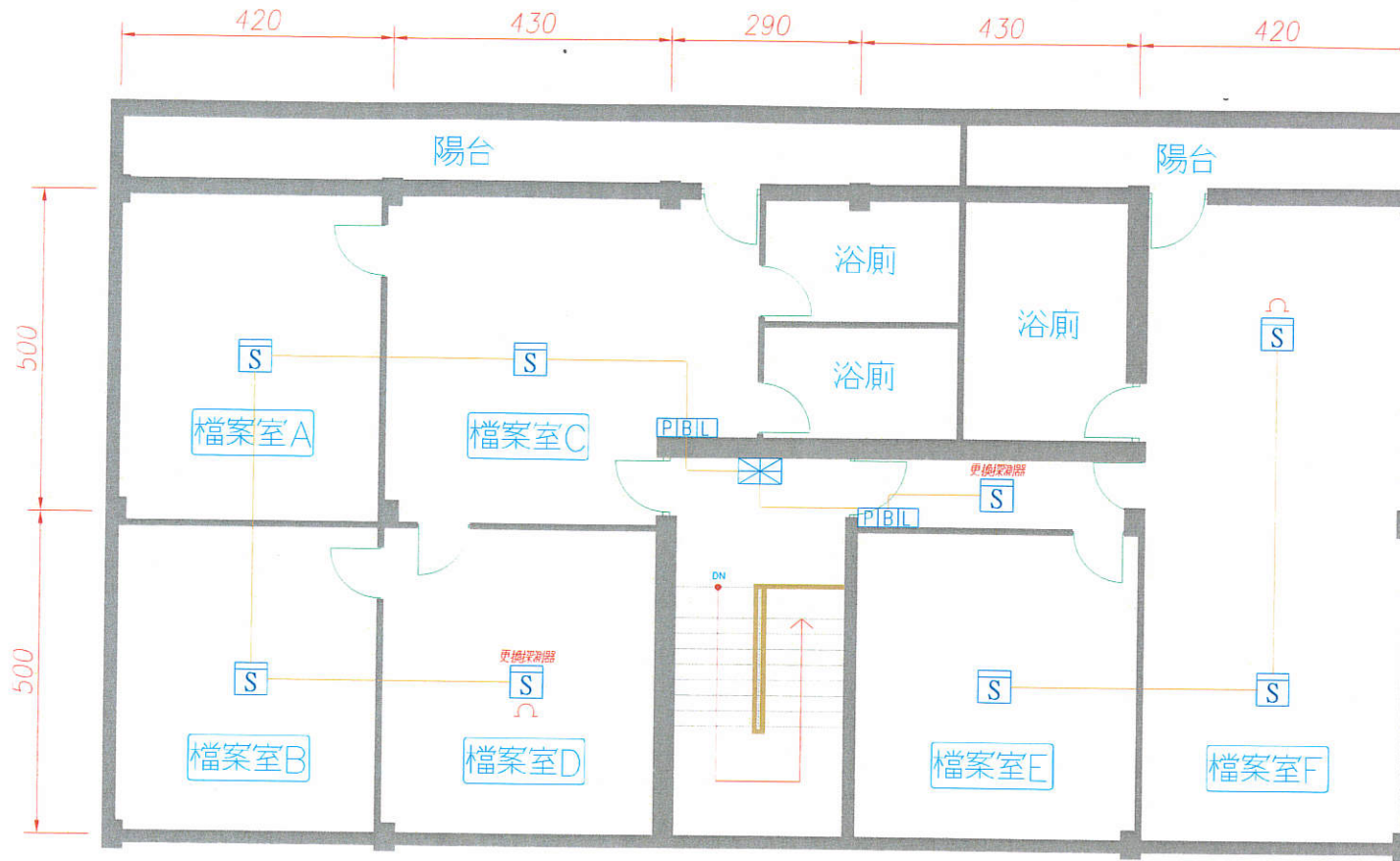
檔案室火警系統配置圖
