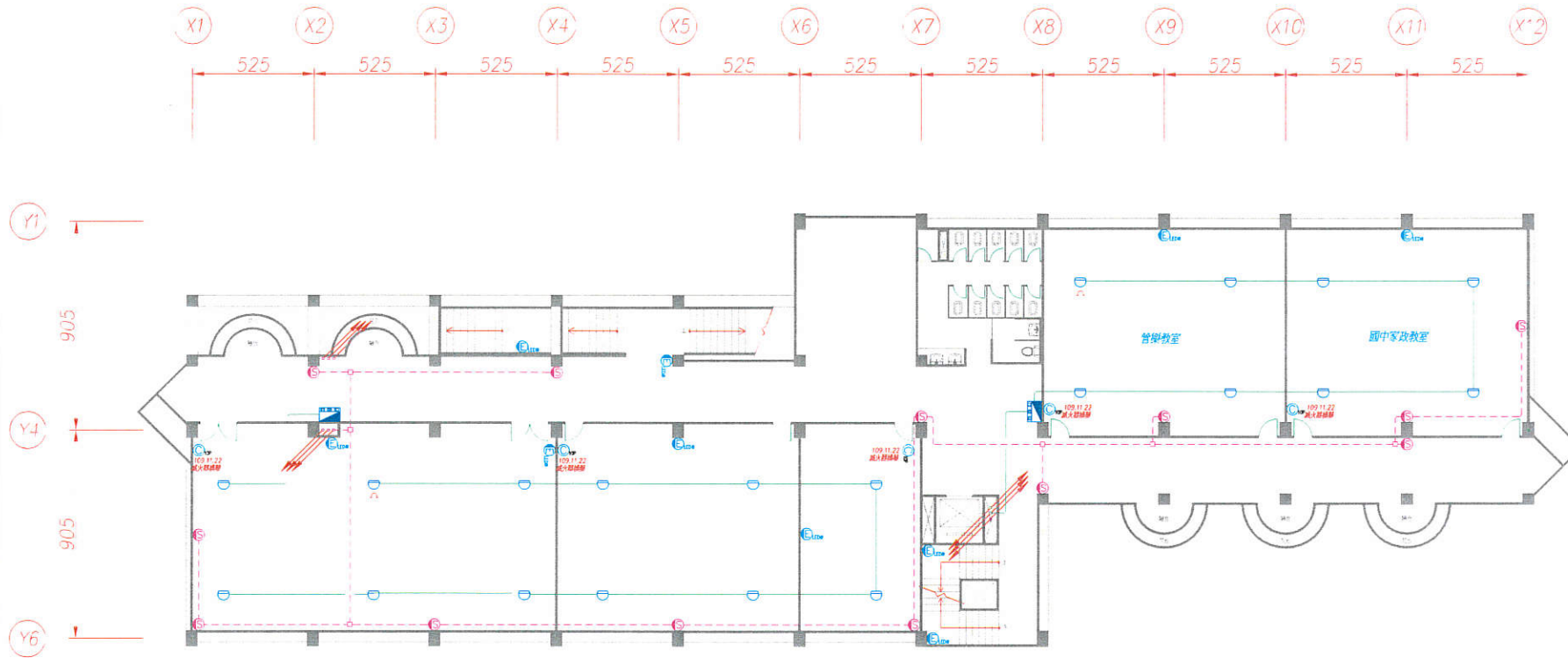
迎曦樓肆樓消防平面圖
