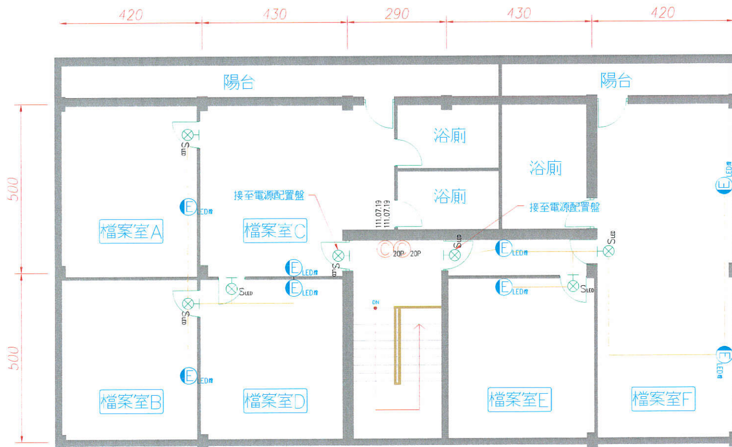
檔案室標示照明, 滅火器配置圖
